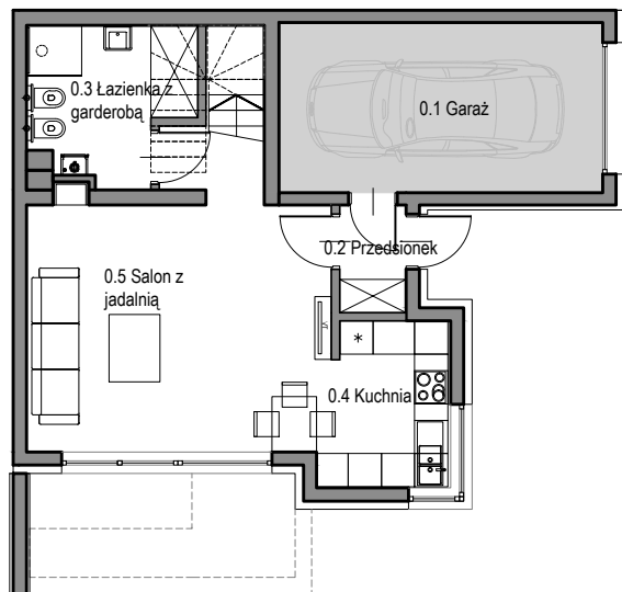
RZUT PARTERU
