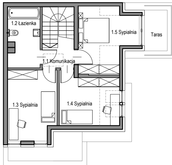
RZUT PODDASZA
